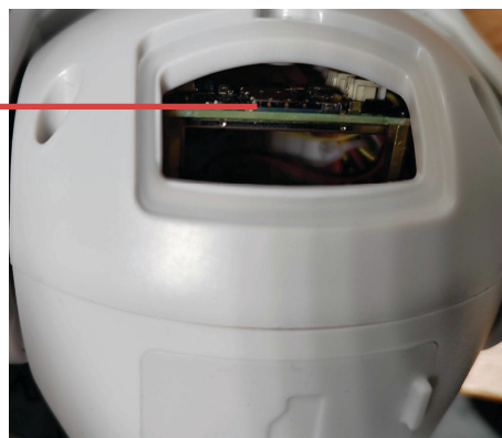
Слот для SIM карты
