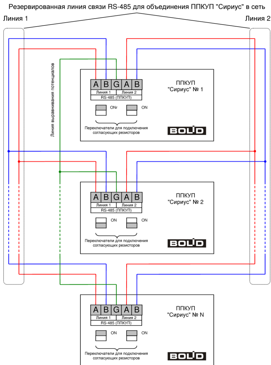
Рисунок 59. Схема объединения приборов «Сириус» в сеть
