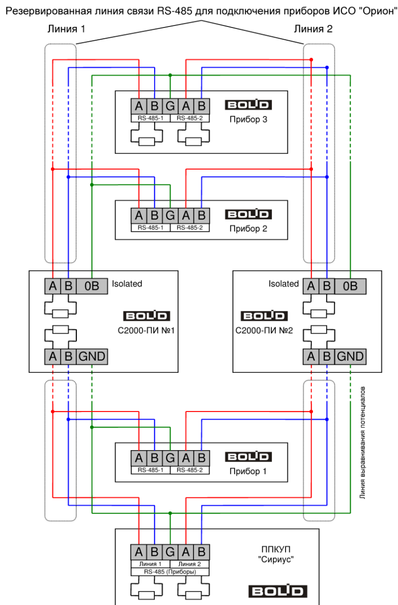
Рисунок 57. Схема подключения повторителей резервированного интерфейса RS-485 «С2000-ПИ»
