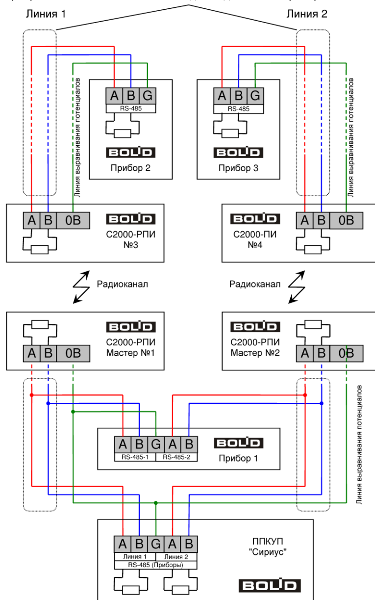
Рисунок 58. Схема подключения преобразователей нерезервированного интерфейса RS-485 «C2000-РПИ»
