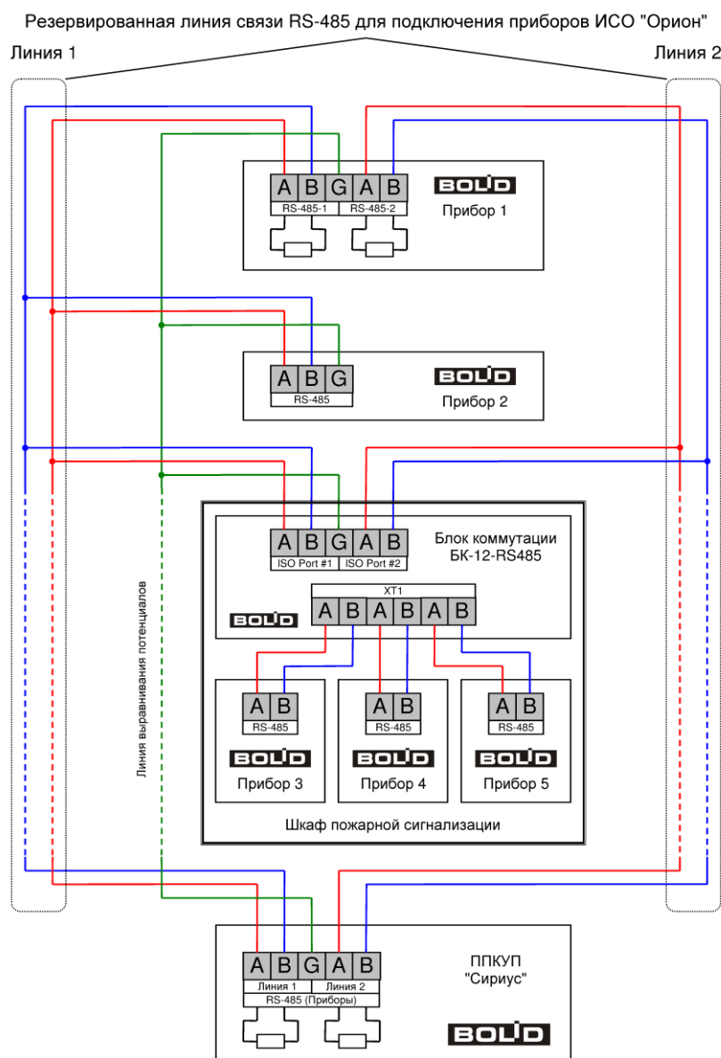
Рисунок 56. Схема подключения дополнительных блоков и приборов ИСО «Орион»
