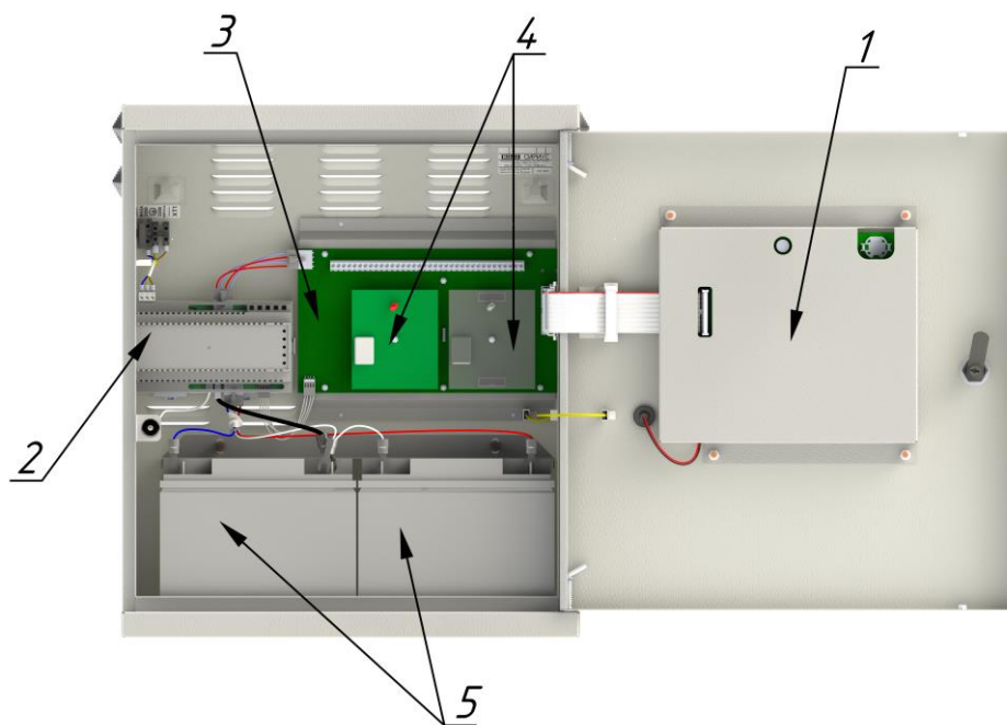
Рисунок 1. Внешний вид прибора (дверь открыта)
