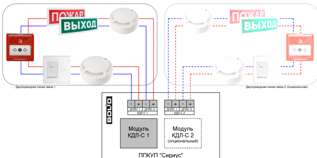
Рисунок 54. Схема подключения адресных устройств
