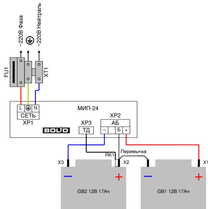
Рисунок 60. Схема подключения источников питания
