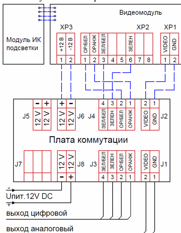
Рисунок 4.3 - Схема подключения термокожуха
