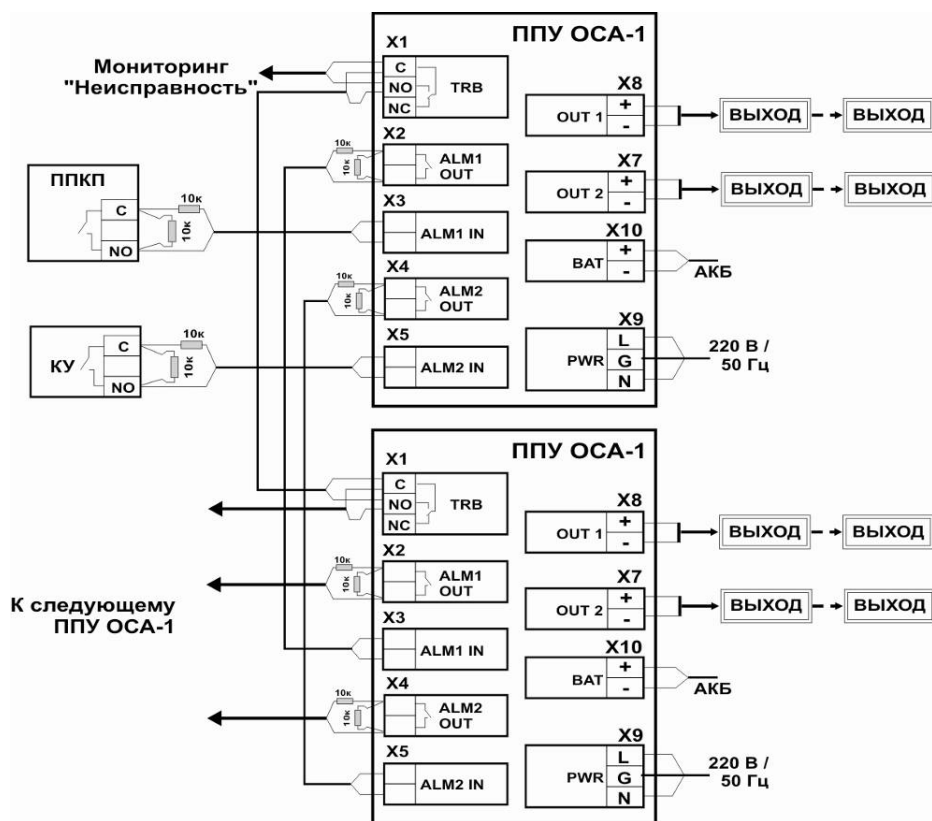
Рис.3б Каскадное соединение нескольких ППУ ОСА-1 (принудительное включение световых табло)
