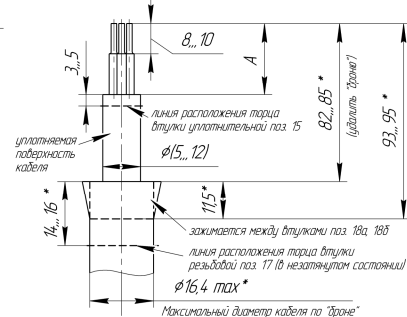
Рис. В.2 – Устройства для крепления защитной оболочки кабеля
