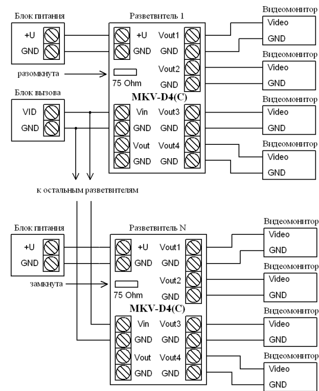
Рисунок 1. Схема подключения разветвителя MKV-D4(C).
