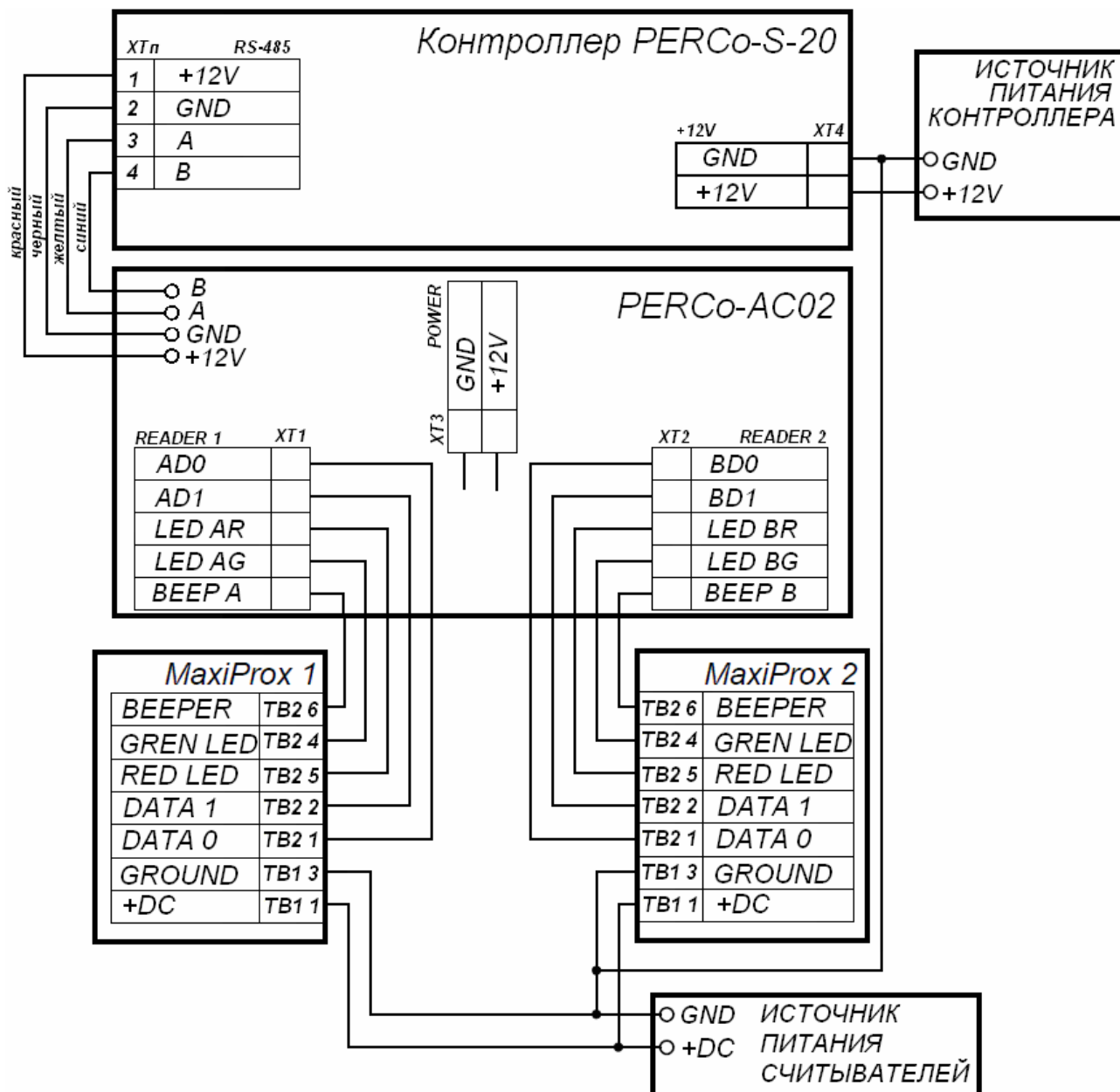
Рисунок 2 Схема подключения считывателя увеличенной дальности HID MaxiProx к контроллеру PERCo-CT/L04
