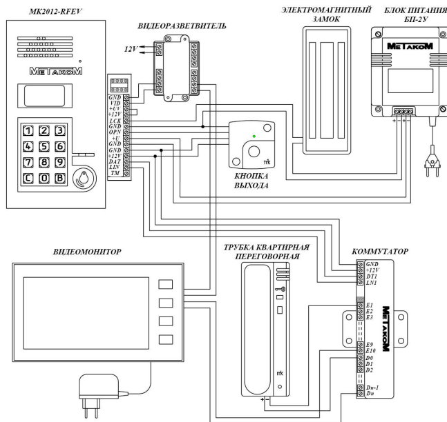
Рис. 2 Пример монтажа блока вызова МК2012-RF(MF)EV
